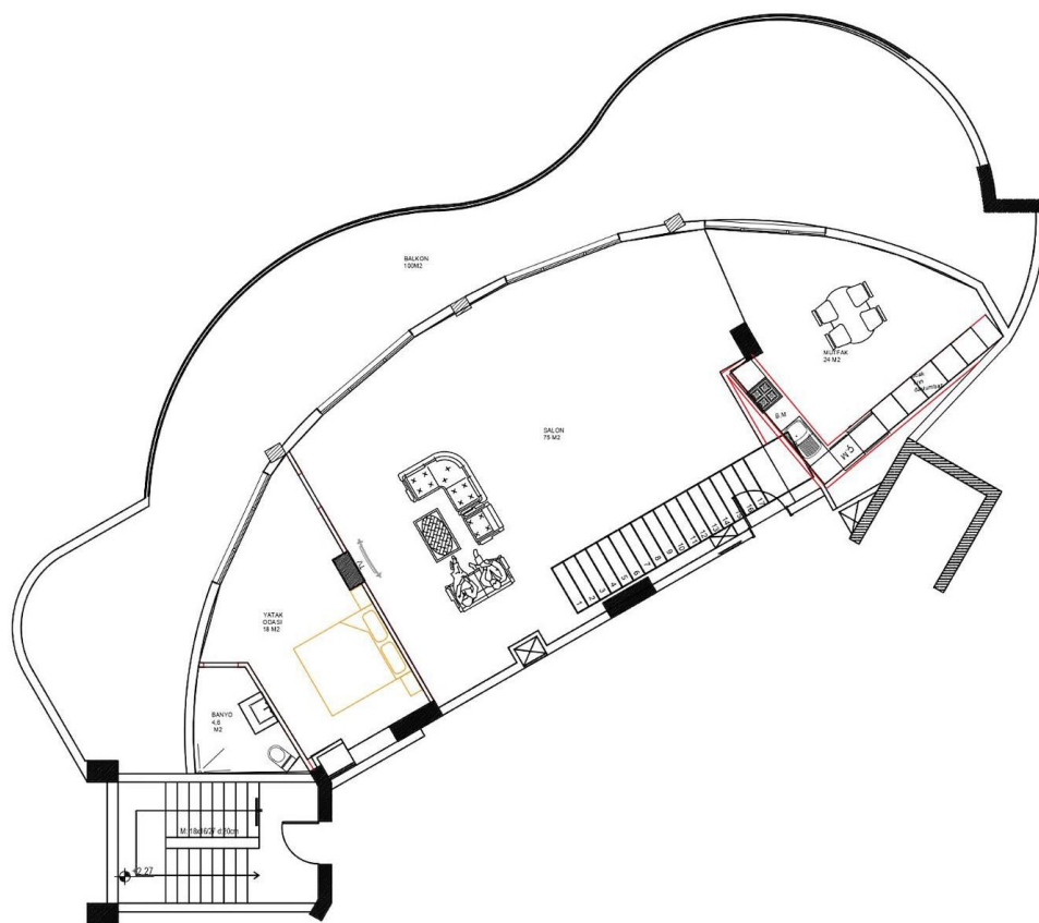
d blok 10 kat nenthouse üst kat
