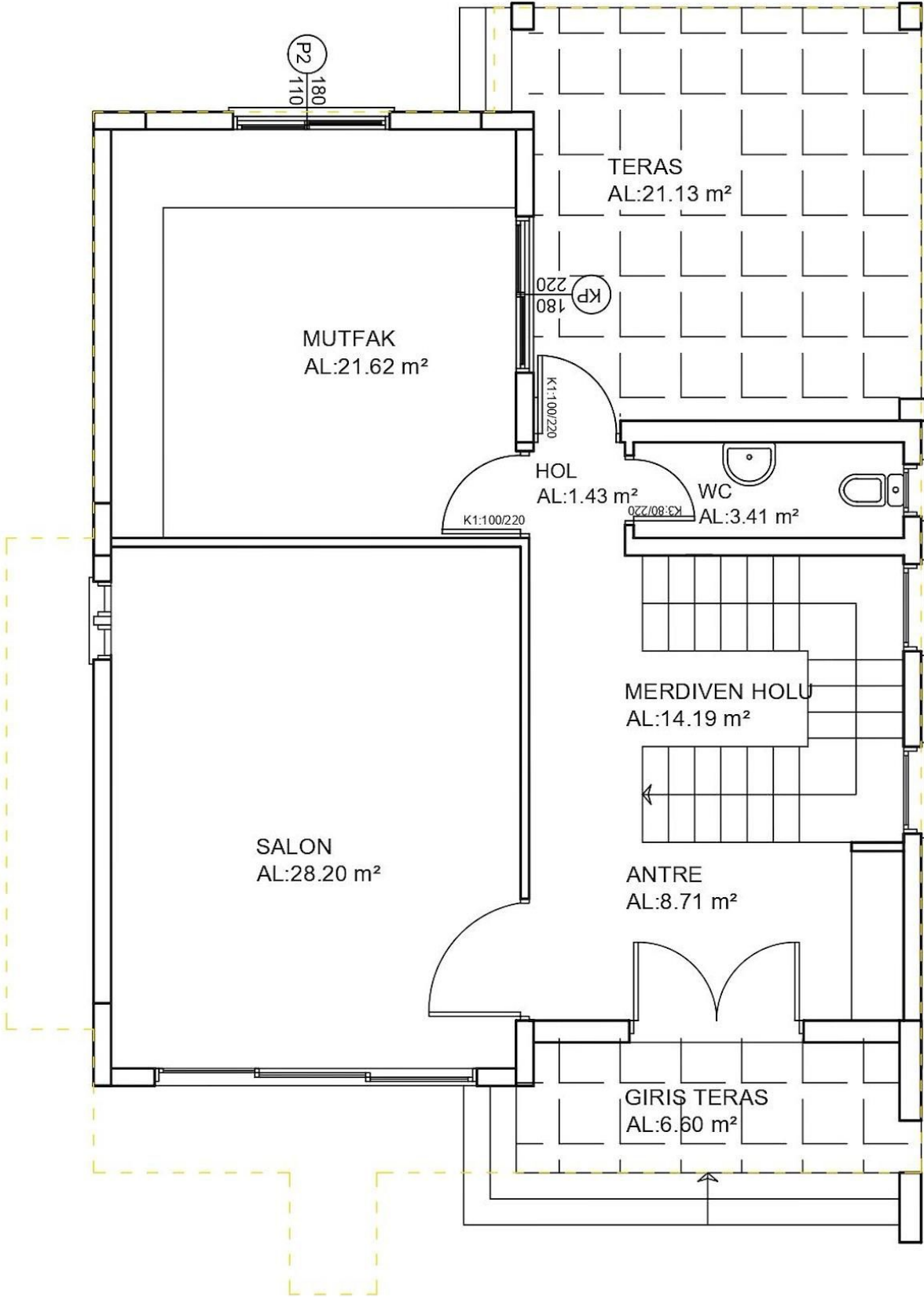
ZEMIN KAT 4+1
