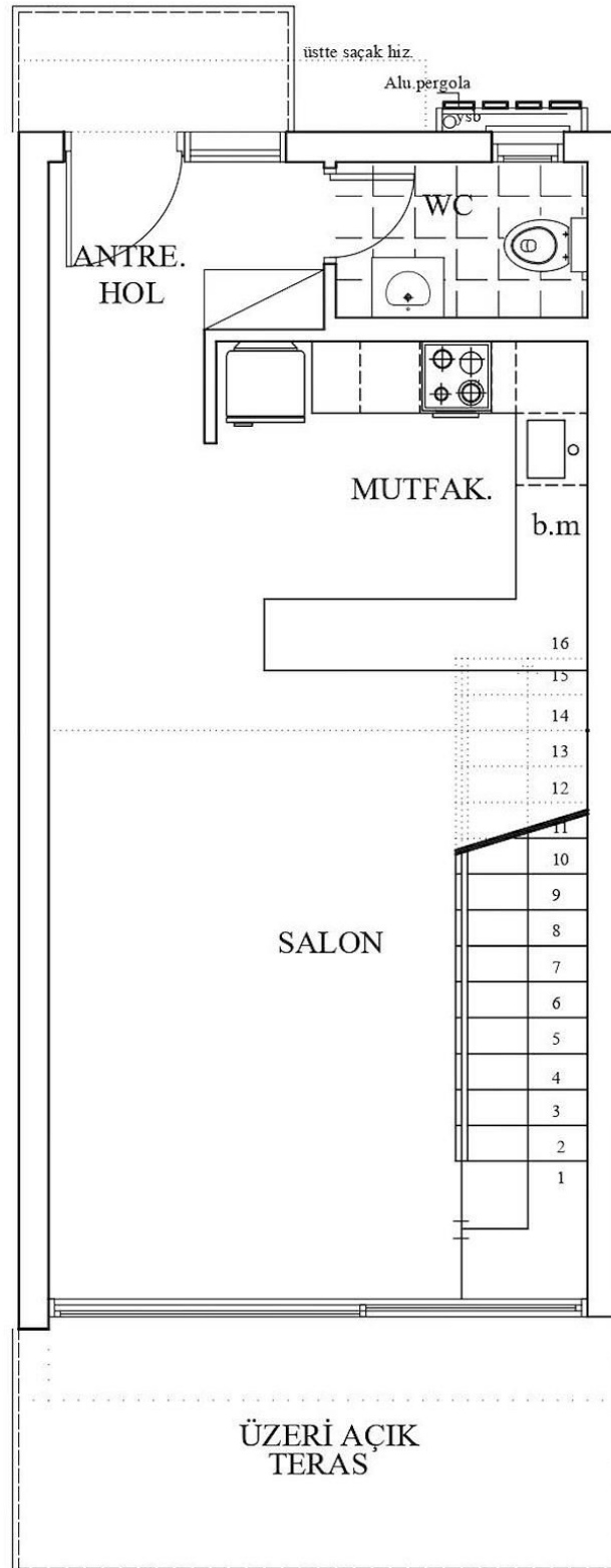
AKOL ESENTEPE F BLOK ZEMİN KAT PLANI
