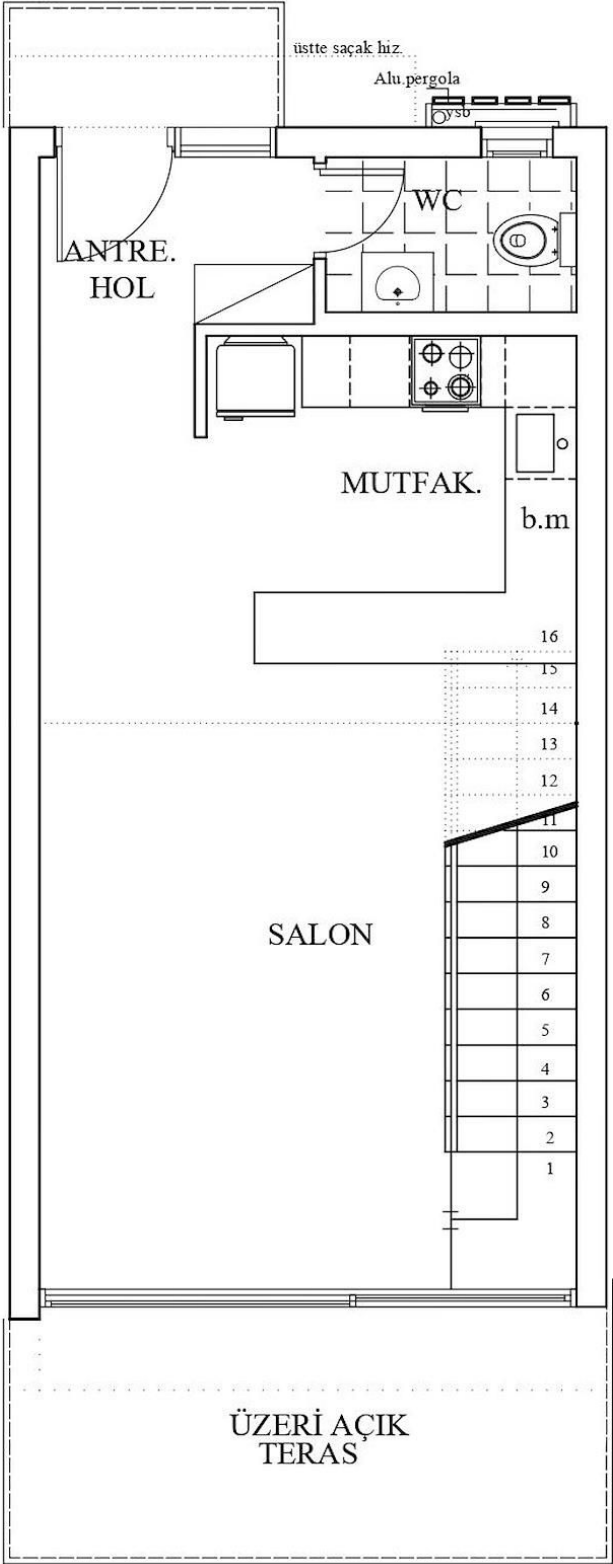
AKOL ESENTEP F BLOK ZEMİN KAT PLANI
